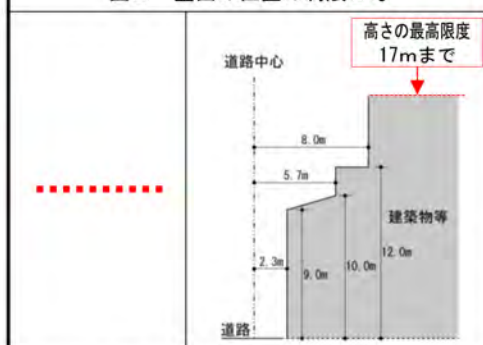
図3 壁面の位置の制限3号
