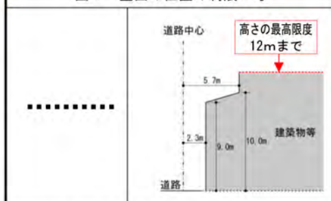
図2 壁面の位置の制限2号
