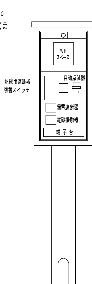
盤内配置図
