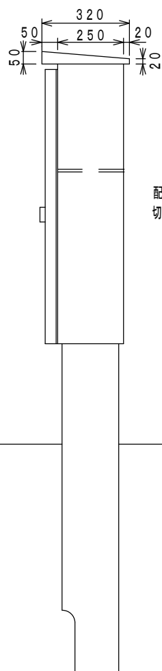
盤姿図（側面）
