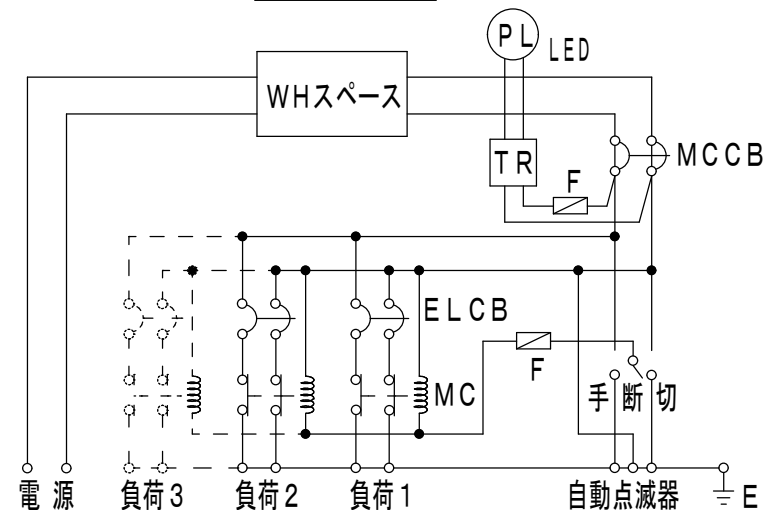
結 線 図
