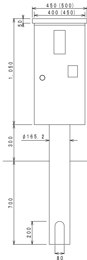
盤姿図（正面）
